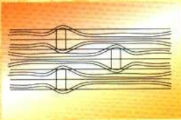
铁心接缝 磁通分布图
